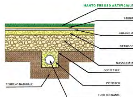
Rappresentazione di un fondo a drenaggio verticale
